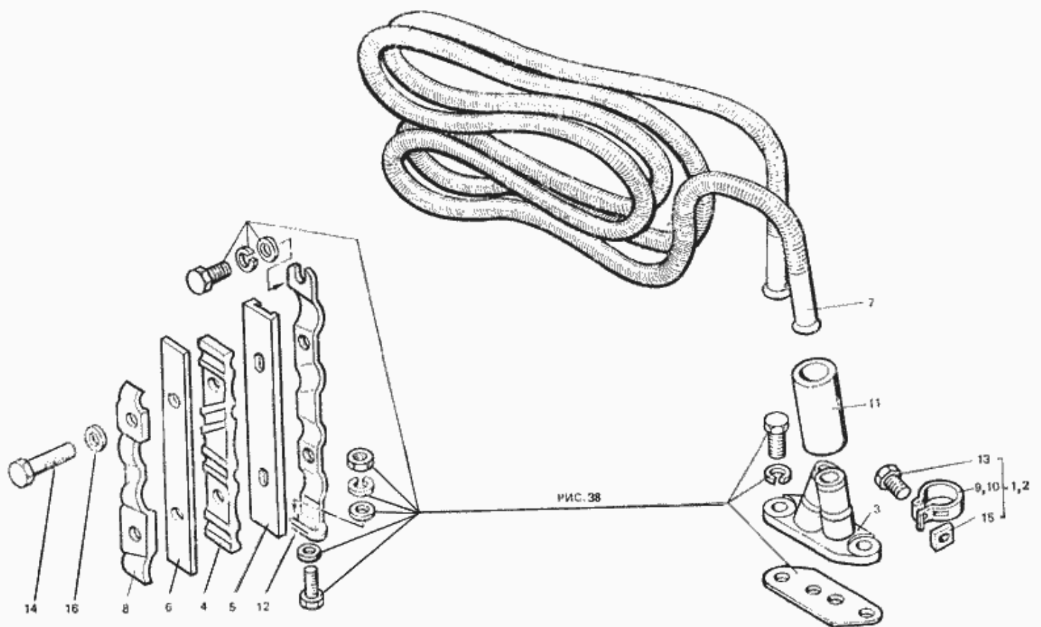
Рис. 40. Радиатор масляный Д144-1405020
